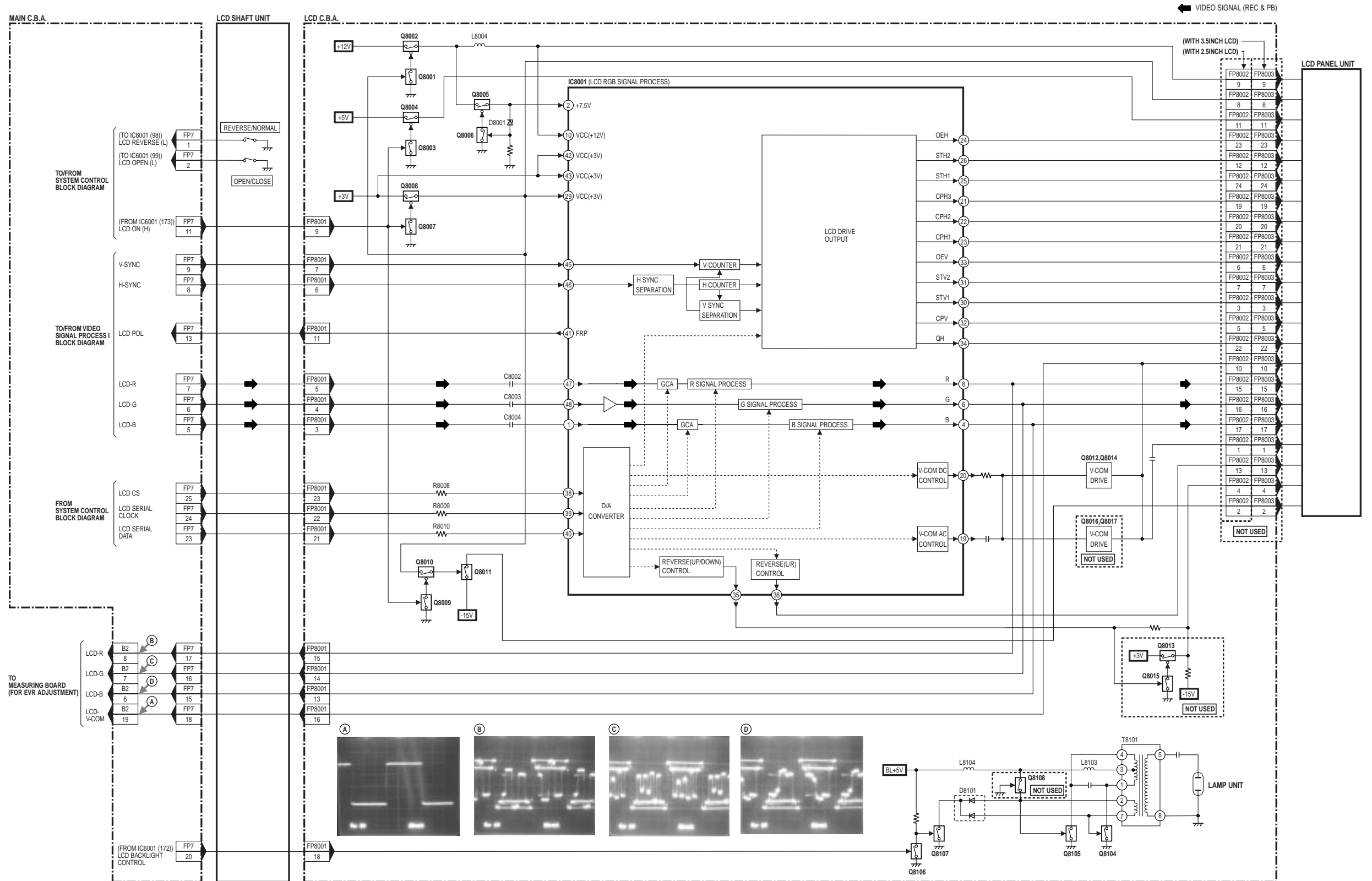
LCD BLOCK DIAGRAM NV-DS29EG/NV-DS29EGM/NV-DS29B/NV-DS29EGE/NV-DS30EG/NV-DS30EGM/NV-DS30B/NV-DS30EGE/NV-DS30EN/NV-DS30ENT/NV-DS30ENC/NV-DS30A/NV-DS50EN/NV-DS50ENT/NV-DS50A
